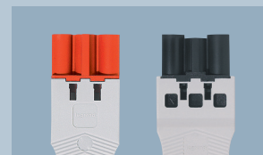
Stekkers met kleurcode om het onderscheid te maken tussen de kringen
